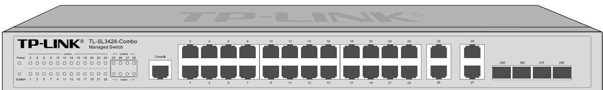
图 2-12 TL-SL3428-Combo 的前面板
