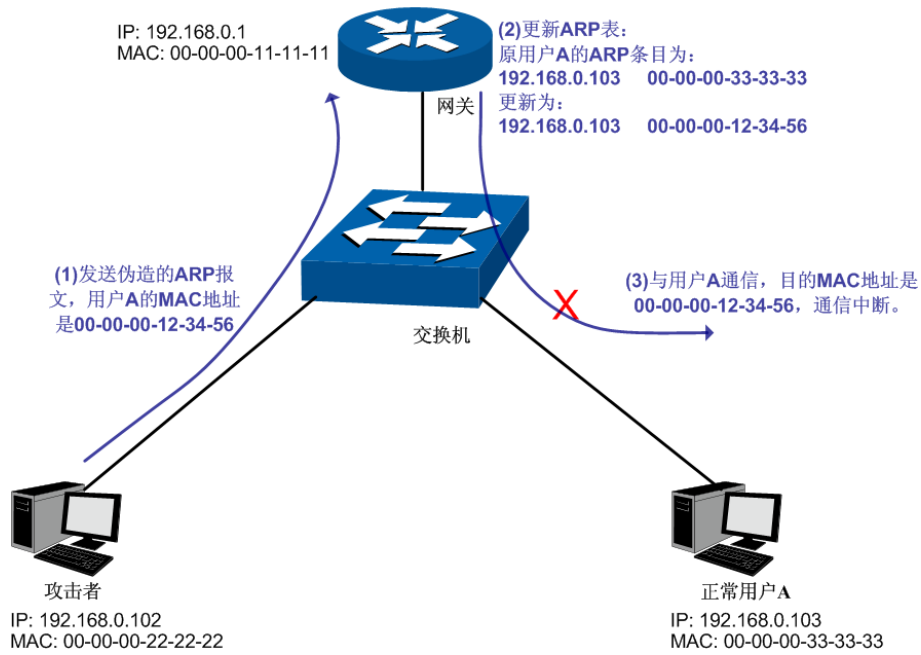
图 12-12 ARP 攻击-欺骗网关示意图
