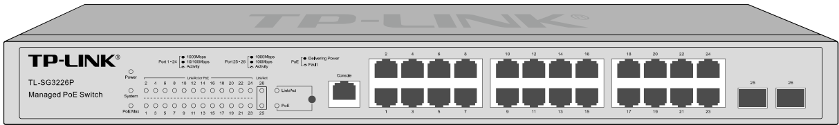
图 2-8 TL-SG3226P 的前面板
