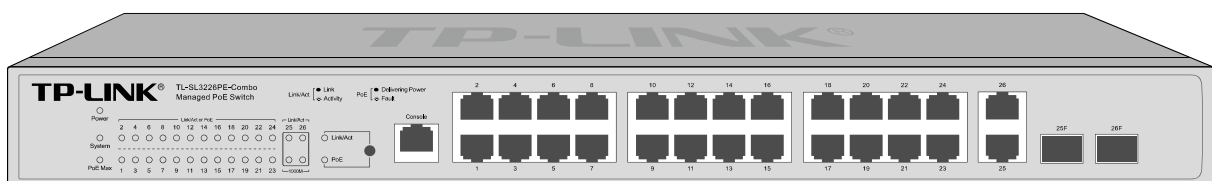
图 2-19 TL-SL3226PE-Combo 的前面板
