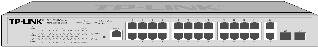
图 2-20 TL-SL3226P-Combo 的前面板
