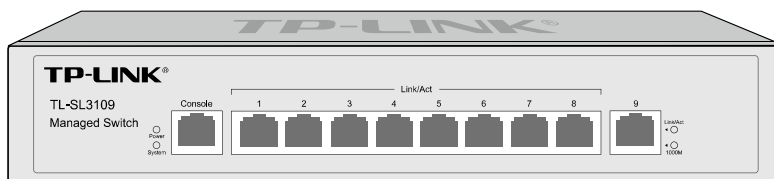
图 2-18 TL-SL3109 的前面板
