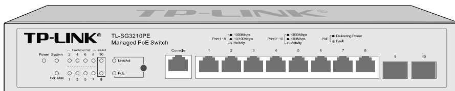
图 2-10 TL-SG3210PE 的前面板
