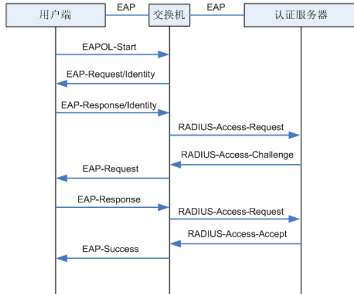
图 12-21 EAP-MD5 认证过程
