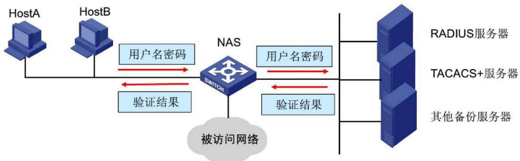
图 12-25 AAA 架构
