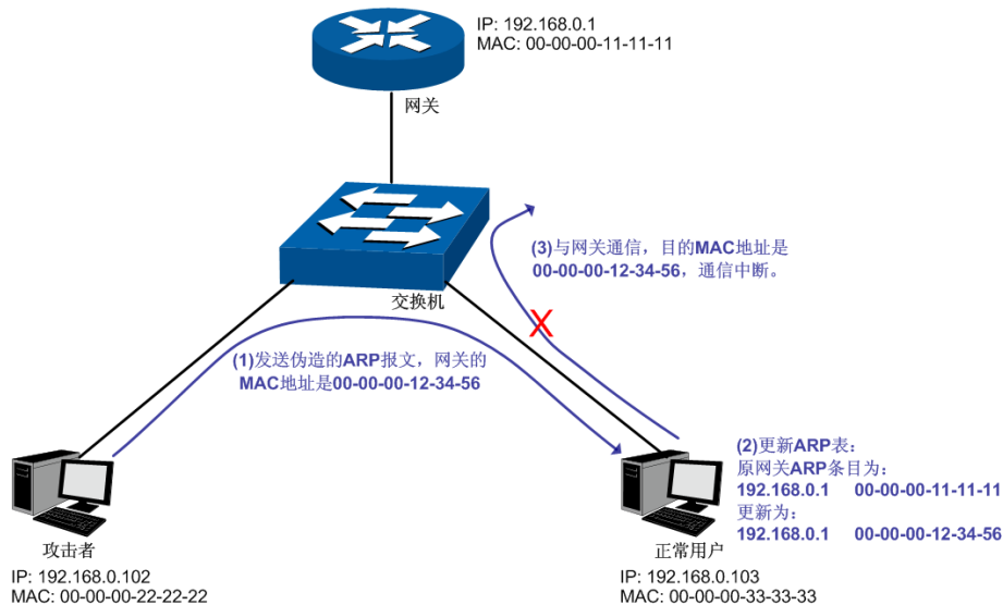
图 12-11 ARP 攻击-网关仿冒示意图
