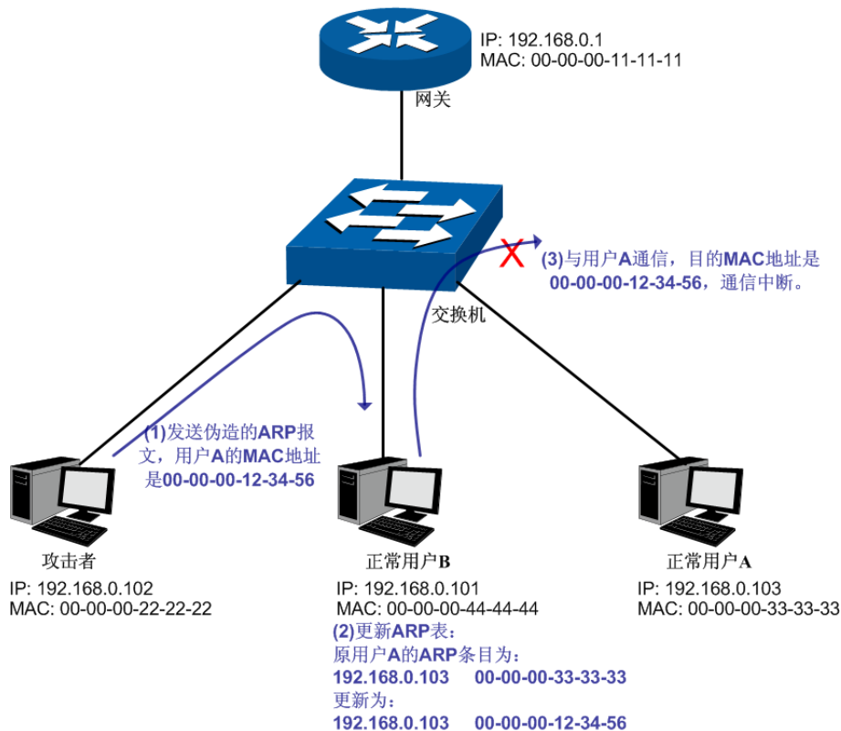
图 12-13 ARP 攻击-欺骗普通用户示意图
