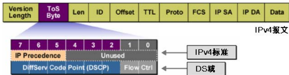
图 9-3 IP 报文
