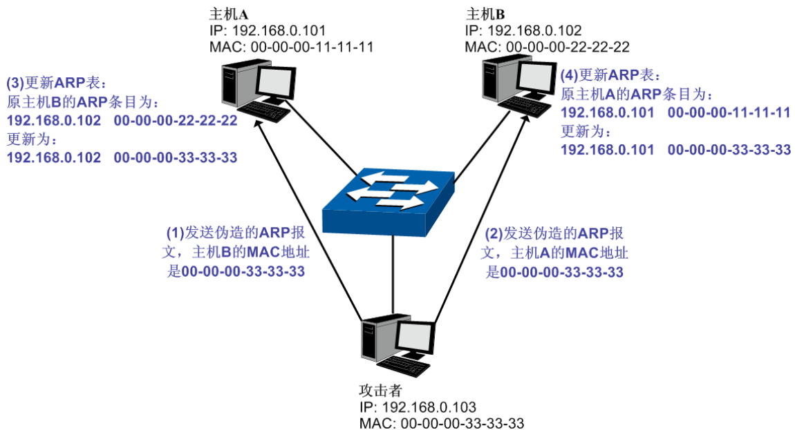
图 12-14 中间人攻击
