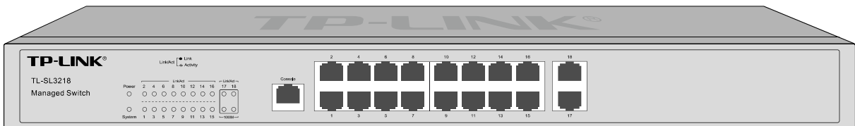
图 2-16 TL-SL3218 的前面板
