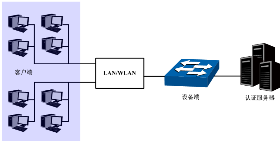
图 12-20 802.1X 认证的体系结构
